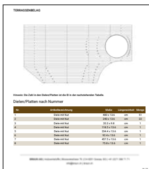
Terrassenbelag Alle Dielenmasse und Mengenangaben in der Übersicht.
