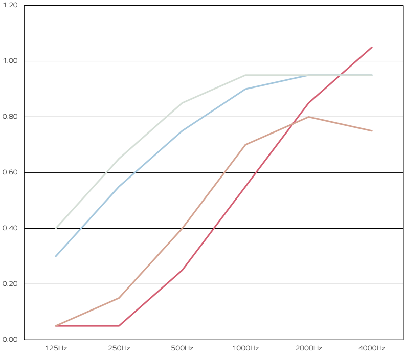
Schallabsorptionskoeffizient ( \alpha_s ) nach EN ISO 354 Universität Stuttgart – Institut für Akustik und Bauphysik IABP
