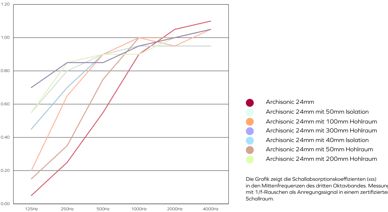
Schallabsorptionskoeffizient ( \alpha_s ) nach EN ISO 354 Universität Stuttgart – Institut für Akustik und Bauphysik IABP
