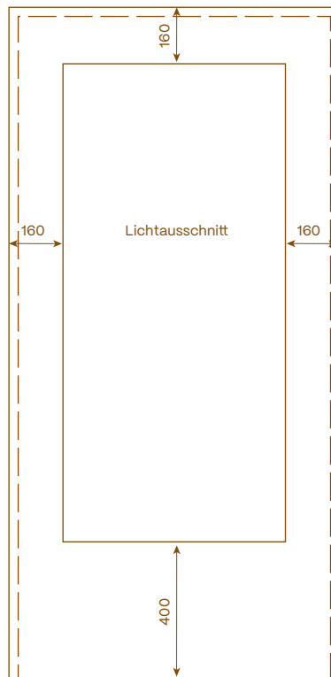
Vollspantür mit Lichtausschnitt
