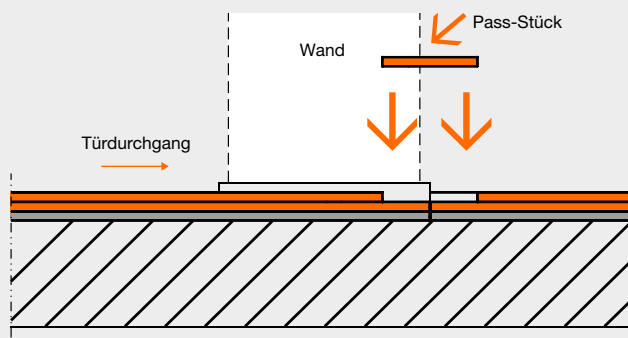
2. In geeigneter Länge, Breite und Dicke einen Streifen aus einer fermacell® Gipsfaserplatte ausschneiden. fermacell™ Estrichkleber auf den Falz auftragen und anschliessend das Pass-Stück einsetzen
