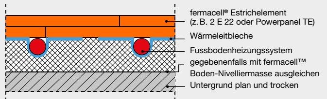
Beispiel 1: fermacell® Gipsfaser Estrichelement 2 E 22 oder Powerpanel TE auf Warmwasser-Fussbodenheizung
