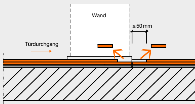
1. Je Seite einen \geq 50 mm breiten Streifen aus fermacell® Gipsfaserplatte von der oberen Lage ausschneiden, z. B. mit einer Handkreissäge
