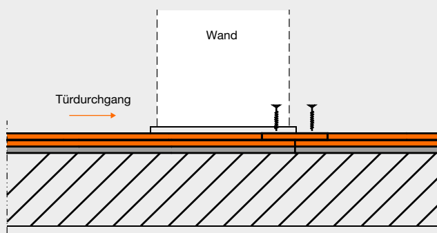
3. Streifen aus fermacell® Gipsfaserplatte und Estrichelement kraftschlüssig miteinander verbinden, z. B. mit fermacell™ Schnellbauschrauben oder Spreizklammern. Der Abstand der Verbindungsmittel darf max. 150 mm betragen
