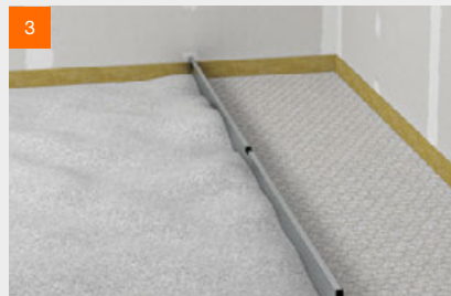
fermacell™ Wabenschüttung abziehen
