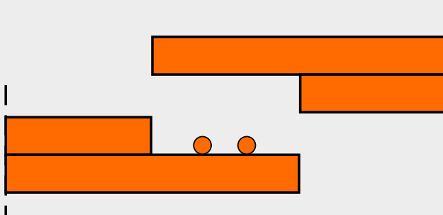
Klebeschnüre ca. 5 mm Ø
