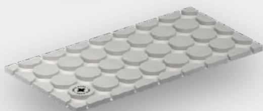
fermacell® Therm25™-125 Element, rund mit Nutabstand 125mm
