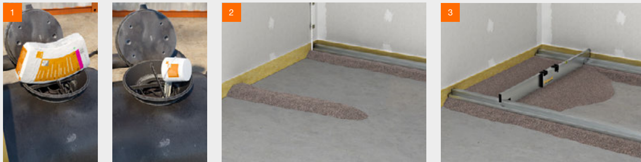
Mischungsverhältnis: 6 Säcke fermacell™ Wabenschüttung + 1 Gebinde fermacell™ Schüttungsbinder
