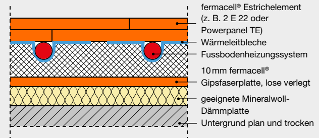
Detail 2: Fussbodenheizungssystem auf zusätzlicher Mineralwoll-Dämmplatte, mit lose verlegter fermacell® Gipsfaserplatte
