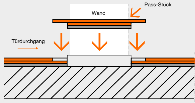
2. Pass-Stück in geeigneter Länge und Breite aus einem fermacell® Estrichelement ausschneiden. fermacell™ Estrichkleber auf den Falz auftragen und anschliessend das Pass-Stück einsetzen
