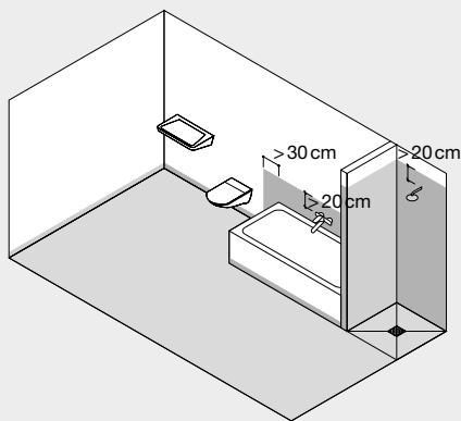
Dusche mit planmässig genutztem Bodenablauf
