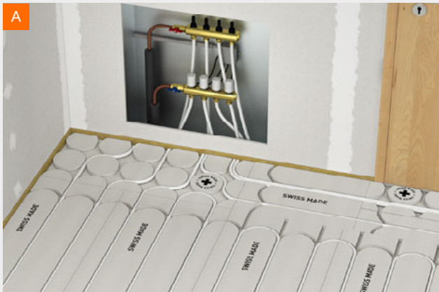
Therm25™ Rund Element vor Heizkreisverteiler mit nachgesägten bzw. nachgefrästen Nuten
