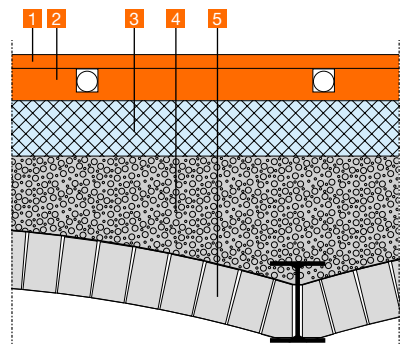
Niveaueinbau auf Gewölbedecke mit fermacell® Therm25™ Element (Bauphysik ist zu beachten)
