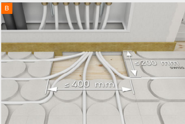
Maximale Größe der Aussparung 400×200mm für Variante 1 beachten.
