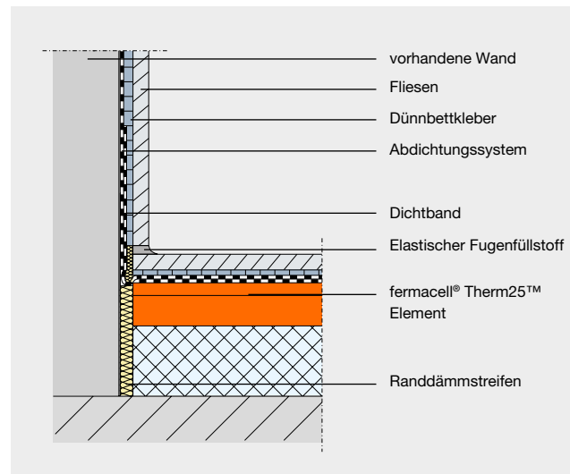
Beispiel: Wand-Fussboden-Anschluss im wasserbeanspruchten Bereich mit fermacell® Therm25™ Element.
