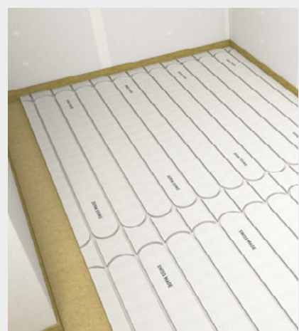
Verlegung der fermacell® Therm25™ Elemente lose verlegt, stumpf gestossen im Kreuzverband
