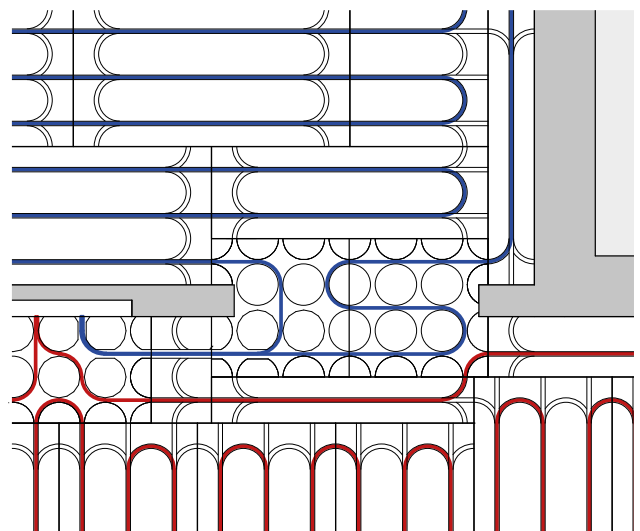
Ausschnitt aus Verlegeschema Tüрдurchgang
