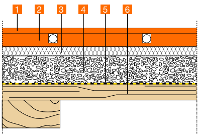
Niveaueinbau auf Holzbalkendecke mit fermacell® Therm25™ Element
