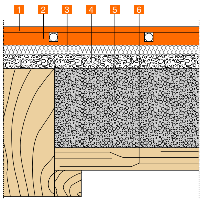
Niveaueinbau der Holzbalkendecke mit tragfähigem Einschub mit fermacell® Therm25™ Element
