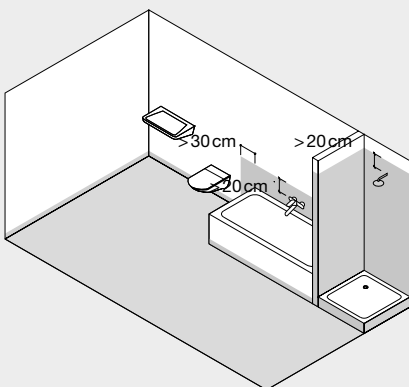
Dusche mit Duschtasse
