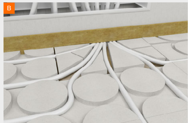
Offen lassen und mit Füllstücken aus fermacell® Gipsfaserplatten ergänzen
